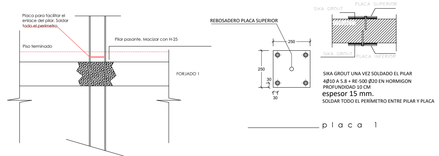
SECCION ENCUESTRO CON FORJADO. BOVEDILLAS
