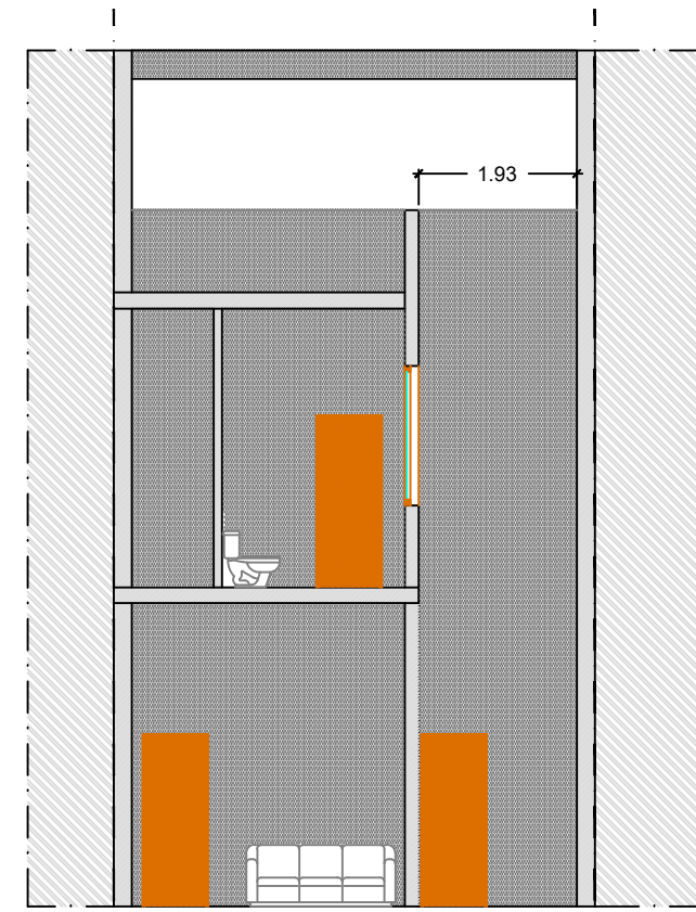
Sección C-C
