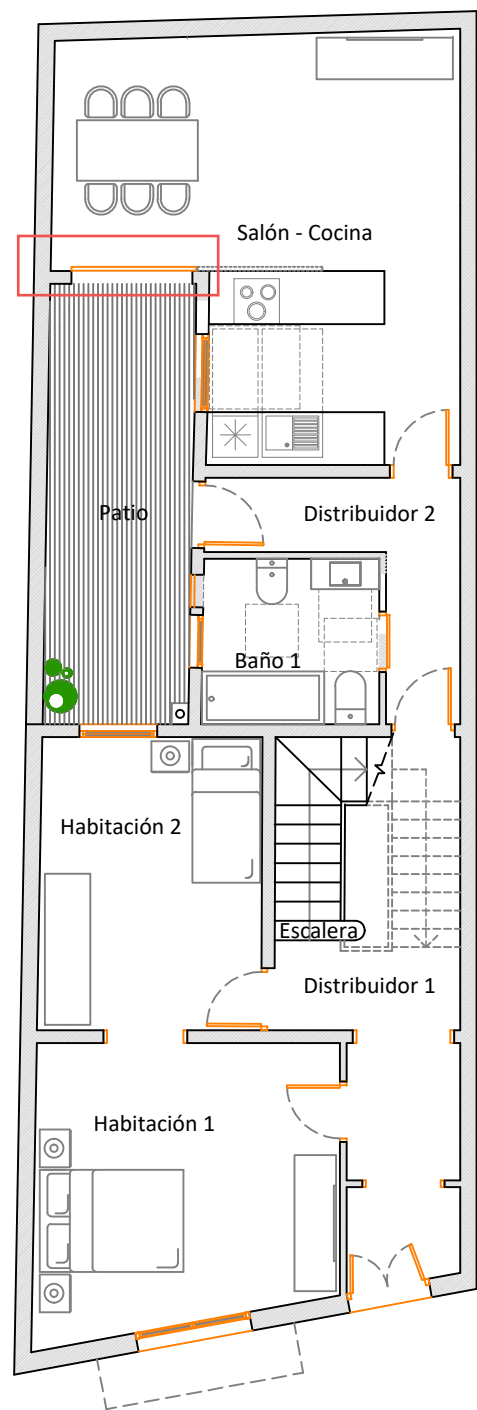
Planta baja
