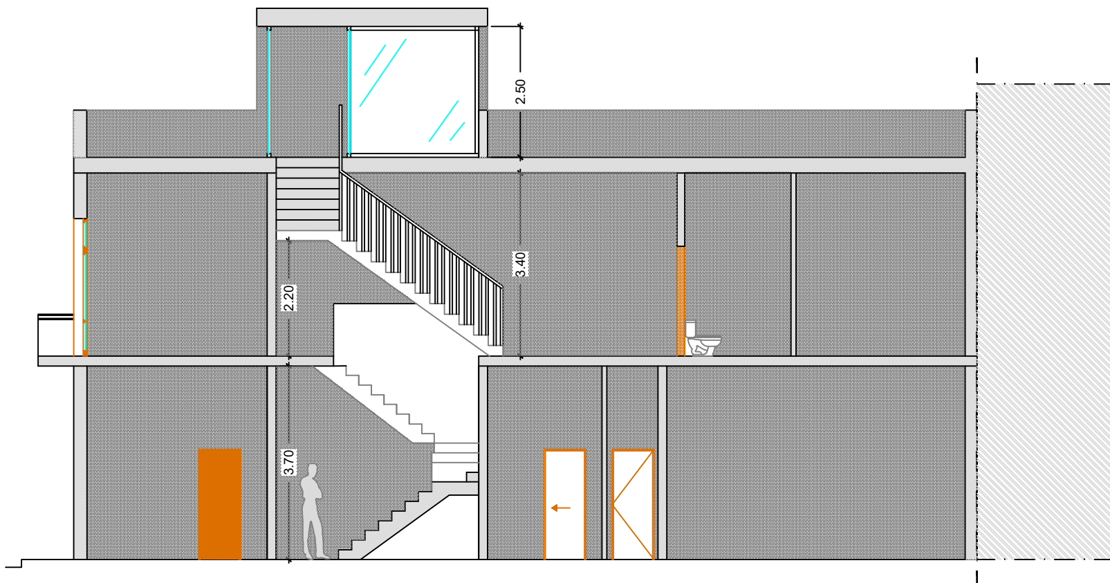
Sección A-A
