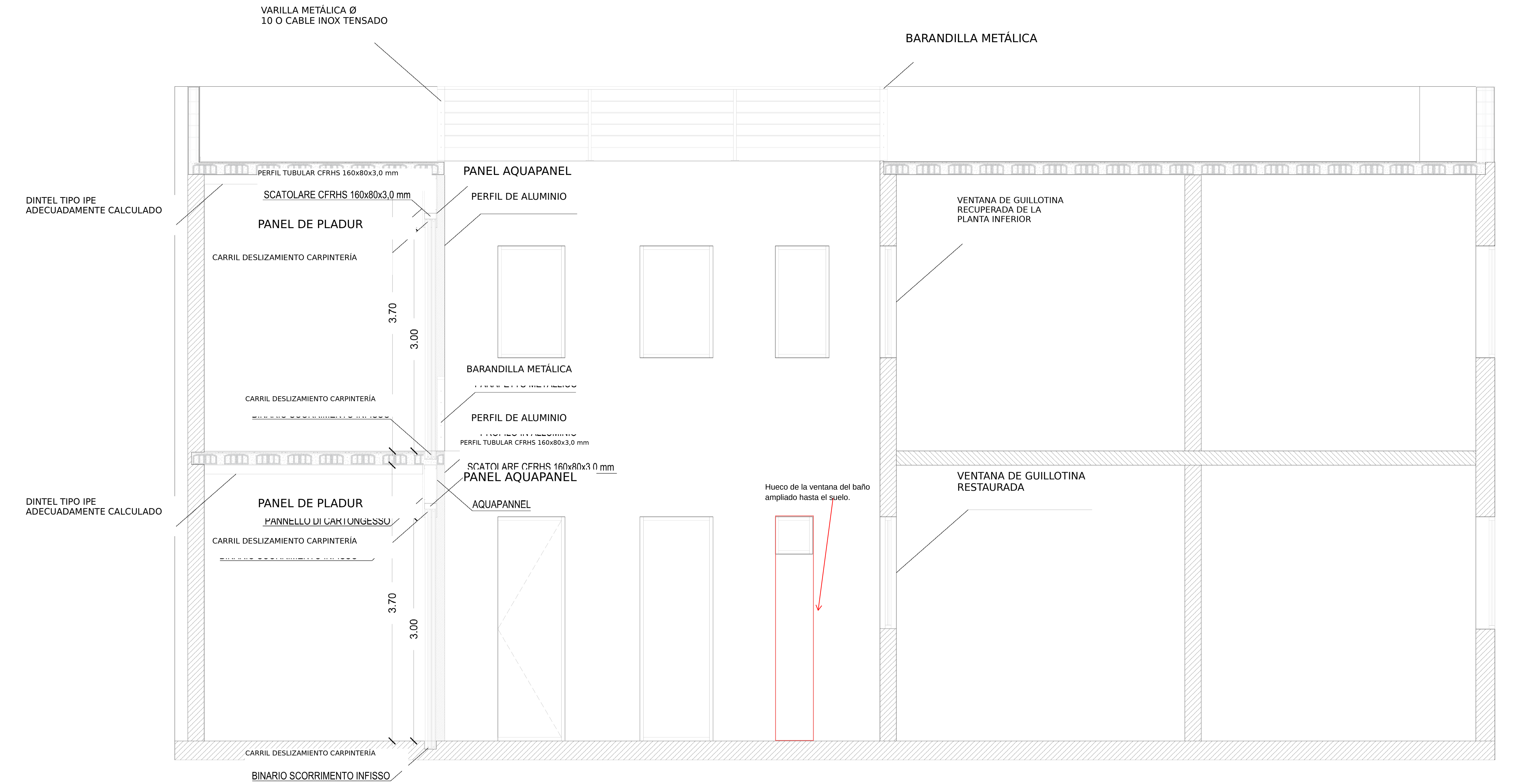
ALZADO OESTE
