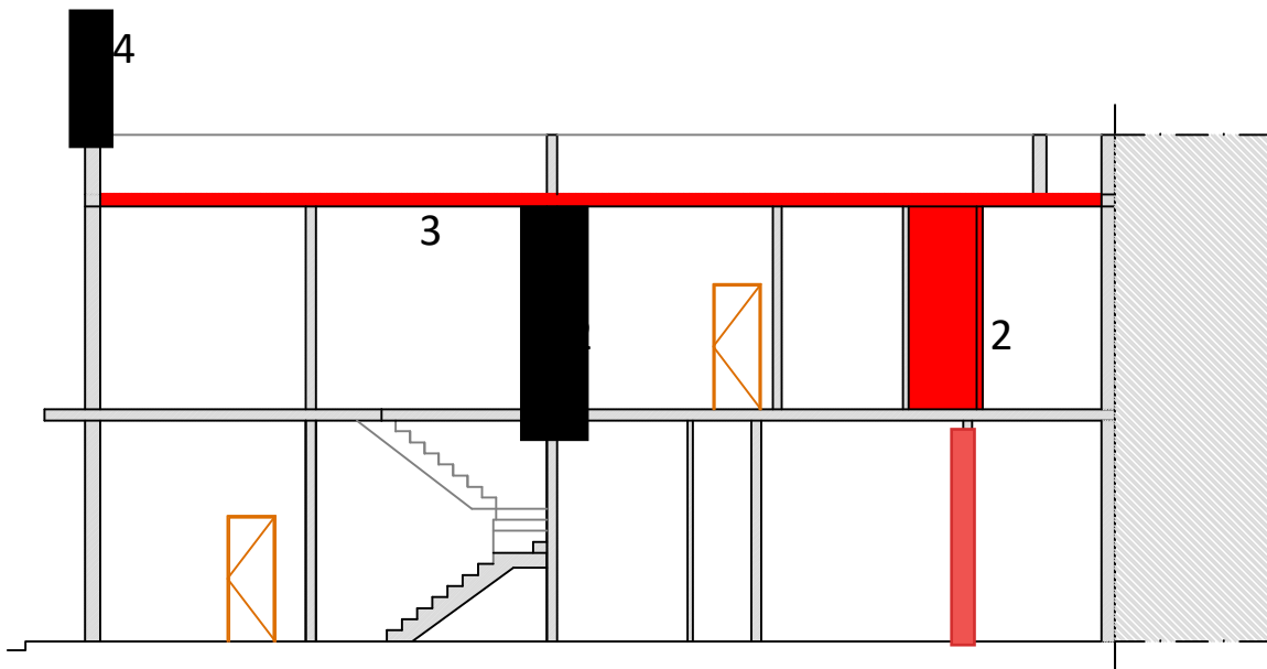
Sección B-B' estado actual con zonas a demoler
