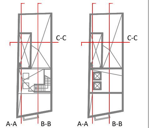
Planta cubierta
